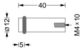
HG 12-40 8,- Möbelknopf mit O-Ring*. Montage mittels M4 Senkkopfschraube.
