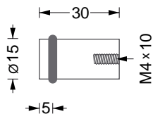
HG 15-30 8,- Möbelknopf mit O-Ring*. Montage mittels M4 Senkkopfschraube.
