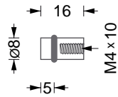
HG 8-16 6,- Möbelknopf mit O-Ring*. Montage mittels M4 Senkkopfschraube.
