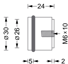
HG 30-24 18,- Möbelknopf mit O-Ring*. Montage mittels M6 Senkkopfschraube.
