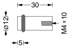
HG 12-30 8,- Möbelknopf mit O-Ring*. Montage mittels M4 Senkkopfschraube.
