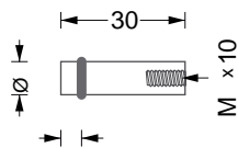
HG 8-30 7,- Möbelknopf mit O-Ring*. Montage mittels M4 Senkkopfschraube.
