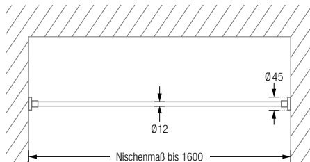
DSN12-1-K45 / -2-K45 Frontansicht:
