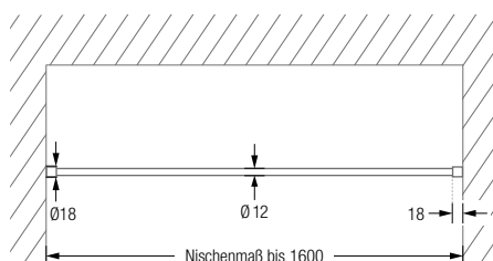
DSN12-1/-2 Frontansicht:
