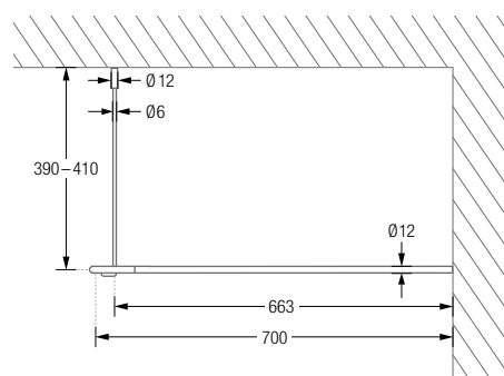
DSU1400-700/1600-700 Seitenansicht:
