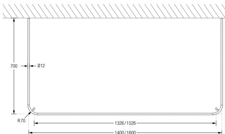
DSU1400-700/1600-700 Draufsicht:
