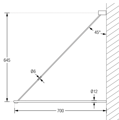
Produktbeispiel DSU1700-700W Seitenansicht:
