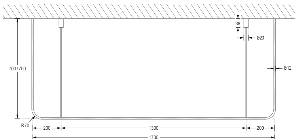
DSU1700-700W / DSU1700-750W Draufsicht:
