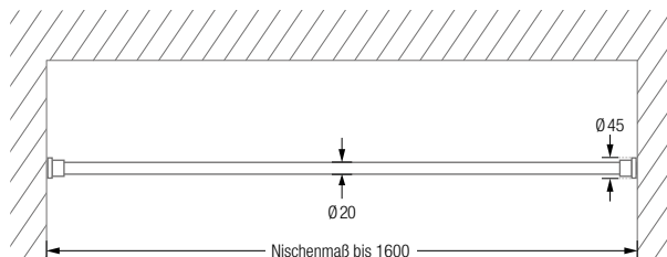
DSRN20-1-K45 / -2-K45 Frontansicht:
