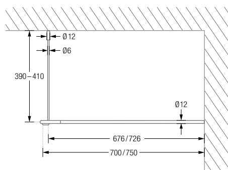
DSU1700-700D/750D Seitenansicht:
