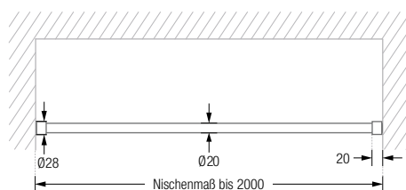
DSRN20-1 / -2 / -3 Frontansicht:
