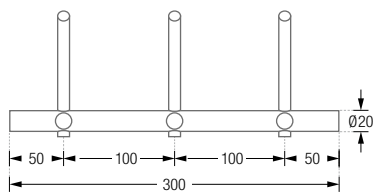
HLS3H Frontansicht:
