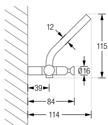
HLS3H / HLS5H Seitenansicht:
