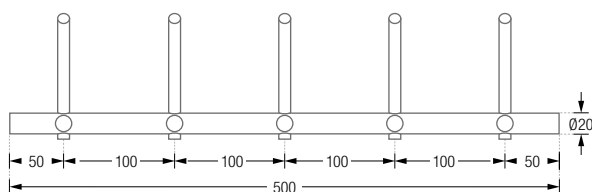
HLS5H Frontansicht:
