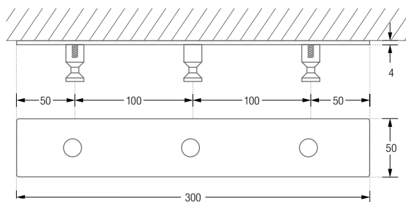
HL3 Drauf- / Frontansicht:
