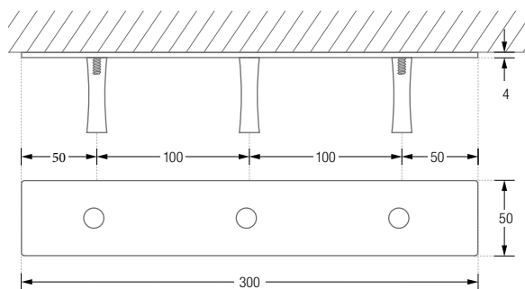
HL3F Drauf- /Frontansicht:
