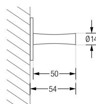
HL3F / HL5F Seitenansicht:
