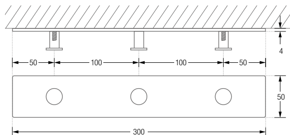
HL3H12S Drauf- /Frontansicht:
