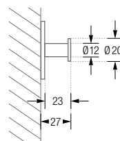
HL3H12S/HL5H12S Seitenansicht:
