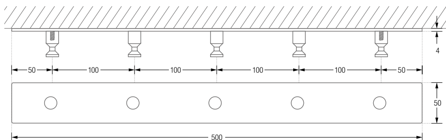
HL5 Drauf- / Frontansicht:
