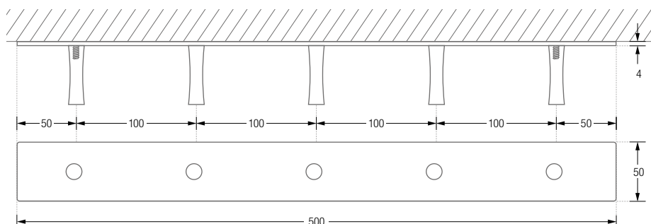
HL5F Drauf- /Frontansicht:
