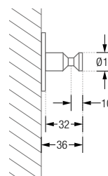
HL3 / HL5 Seitenansicht:
