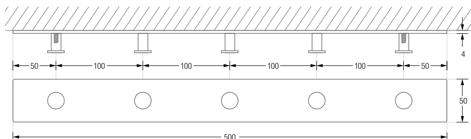
HL5H12S Drauf- /Frontansicht:
