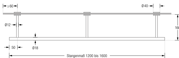
GSUN18-2 Frontansicht:
