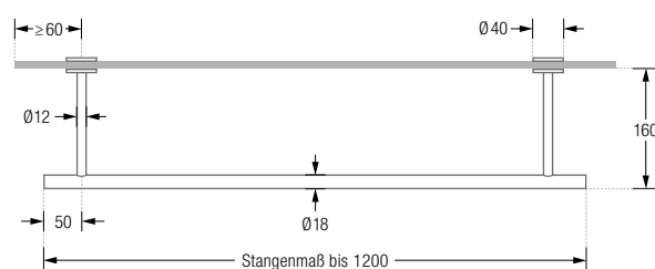
GSUN18-1 Frontansicht:
