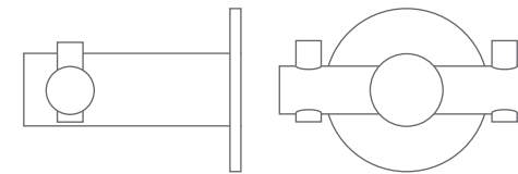
H18-50DR40 Doppel-Haken zur Verschraubung Ø18 mm, Länge 53 mm, Breite 62 mm
