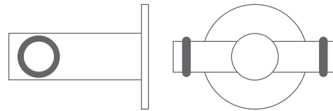
HG18-50DR40 Doppel-Haken zur Verschraubung Ø18 mm, Länge 53 mm, Breite 62 mm
