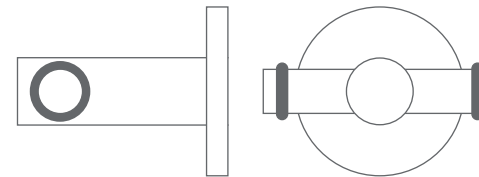
HG18-50DK45 Doppel-Haken zur Verklebung Ø18 mm, Länge 56 mm, Breite 62 mm
