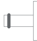
HG12-30K40 zur Verklebung Ø12 mm, Länge 36 mm
