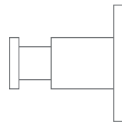
HN20-40K45 zur Verklebung Ø20 mm, Länge 46 mm
