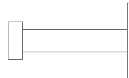
HSF2-L-R40 zur Verschraubung Ø12 mm, Länge 65 mm
