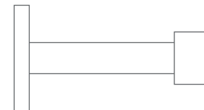
HSF3-L-WS zur Verschraubung Ø12 mm, Länge 75 mm
