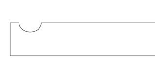
HV18-80R40 zur Verschraubung Ø18 mm, Länge 83 mm
