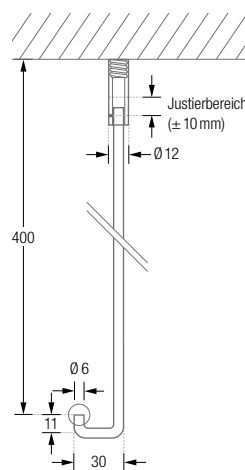
DTD Seitenansicht:
