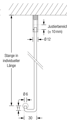
DTDM Seitenansicht:
