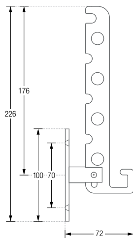
Produktbeispiel KL1 zugeklappt:
