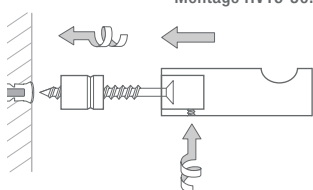
Montage HV16-50:
