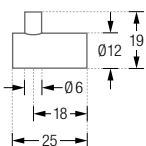
H12-25E:
