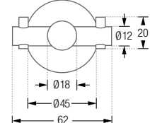
H18-50DK45 Frontansicht:
