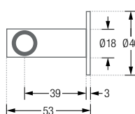
HG18-50DR40 Seitenansicht:
