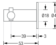
H18-50DR40 Seitenansicht:
