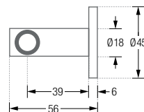
HG18-50DK45 Seitenansicht:
