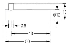
H12-50E:
