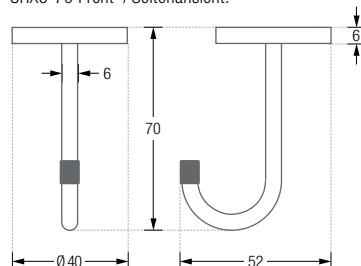
UHX6-70 Front- / Seitenansicht:
