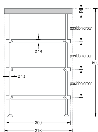
Produktbeispiel SB800-3-Eiche-B Seitenansicht:
