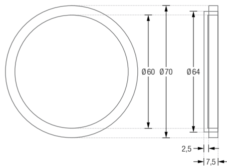
STG70F Front- / Seitenansicht:
