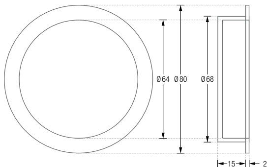
STG80 Front- / Seitenansicht:
