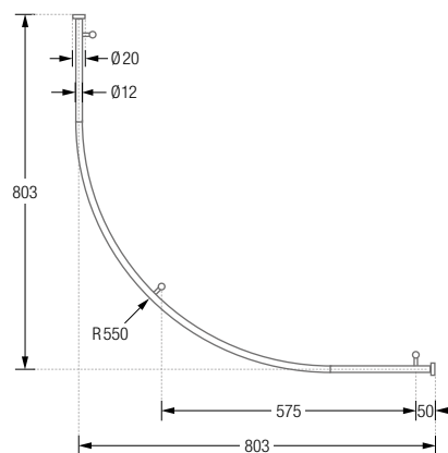
Produktbeispiel DSB550-800F Draufsicht:
