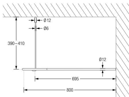
Produktbeispiel DSB300-800 Seitenansicht:
