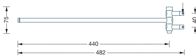
Seitenansicht
