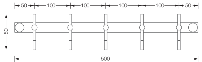
Frontansicht
