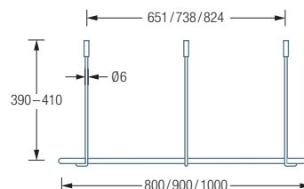
DR800 / 900 / 1000 Seitenansicht:
