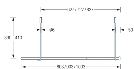
DSB550-800F / 900F / 1000F Seitenansicht:
