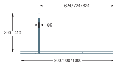
DSB550-800 / 900 / 1000 Seitenansicht:
