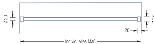
DSRN20 Frontansicht:
