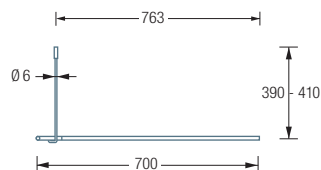
DSU1700-700D-B70 Seitenansicht:
