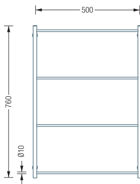
HTL18-500WG Frontansicht:
