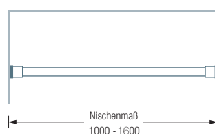
TKS20-2 Frontansicht:
