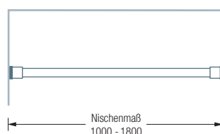
TKS20-2 Frontansicht:
