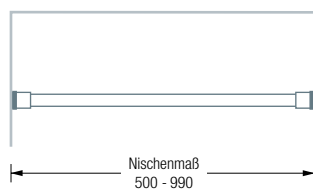
TKS20-1 Frontansicht:
