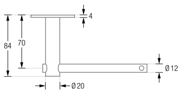
TPH3-140 Draufsicht:
