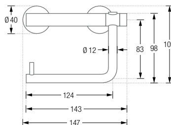
TPH4-K40 Frontansicht:
