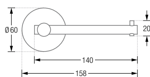
TPH3-140 Frontansicht:
