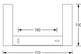
PHA1 Rückansicht:
