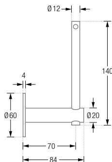
RTPH2-140 Seitenansicht:
