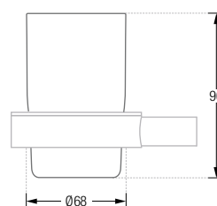
ATGG Seitenansicht:
