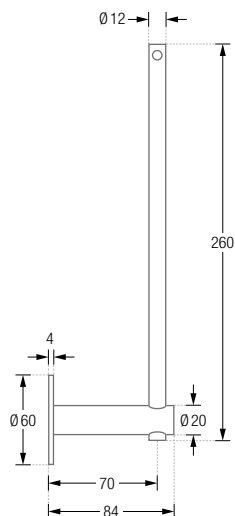
RTPH2-260D Seitenansicht:
