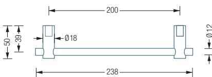
BG12-238 Draufsicht:
