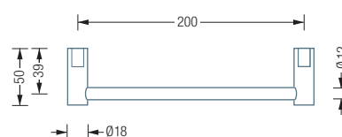
BG12-900E Draufsicht:
