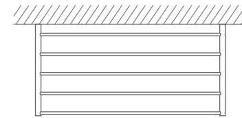
Schuhregal SR600-2W Breite 62 cm, Höhe 22 cm
