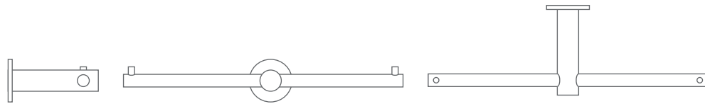
TPH3-260D Seitenansicht/Frontansicht/Draufsicht
