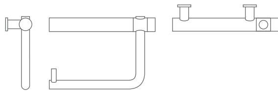
TPH4 Seitenansicht/Frontansicht/Draufsicht
