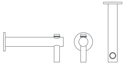
TPH1 Seitenansicht/Frontansicht/Draufsicht
