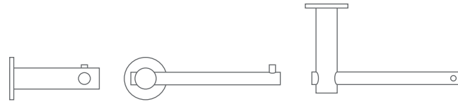
TPH3-140 Seitenansicht/Frontansicht/Draufsicht
