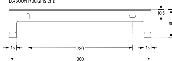
DA300H Rückansicht:
