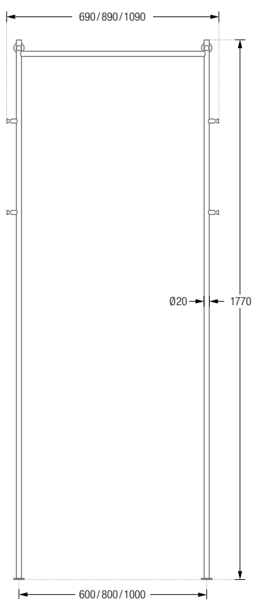
GL2 Frontansicht:
