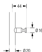
Kleiderhaken mit konischer Nut:
