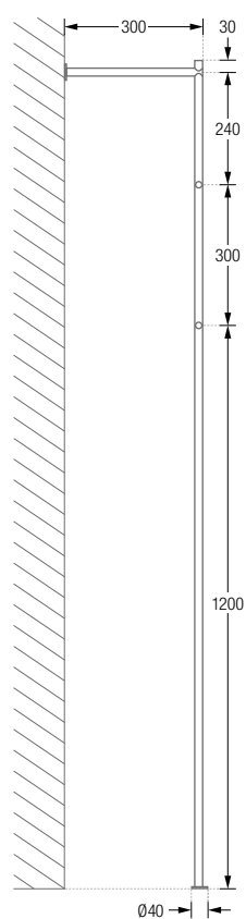
GL2 Seitenansicht:
