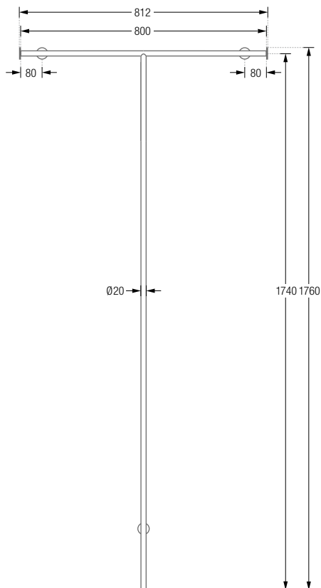
GT1 Frontansicht:
