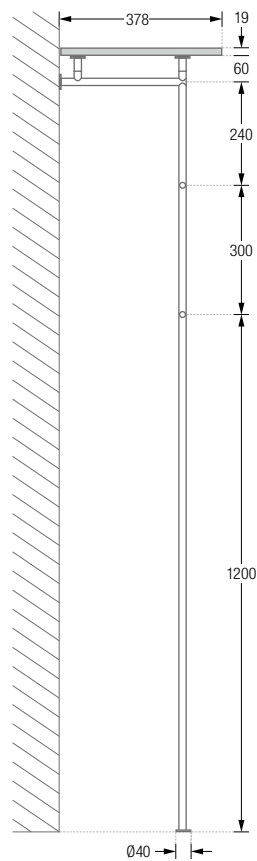
GL2-Eiche Seitenansicht:
