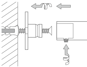
Montage GL2G:
