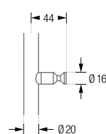
Kleiderhaken mit konischer Nut:
