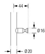
Kleiderhaken mit konischer Nut:
