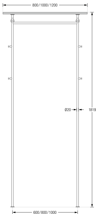
GL2-Eiche Frontansicht:
