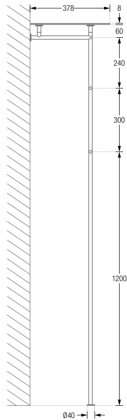
GL2G Seitenansicht:
