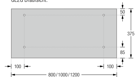
GL2G Draufsicht:
