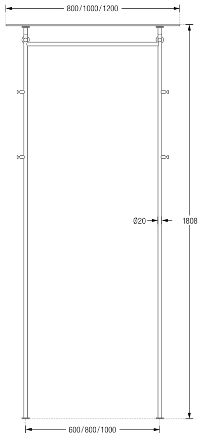
GL2G Frontansicht:
