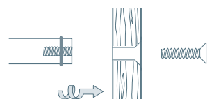
Montage auf Panel, rückseitig verschraubt:
