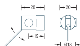
Winkelflexible Wandbefestigung:
