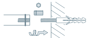
Montage auf Wand:
