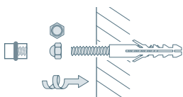
Wandmontage mit Stockschraube:
