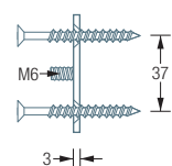
R55S Seitenansicht:
