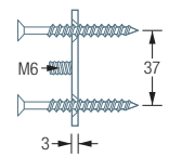
R55VN Seitenansicht:
