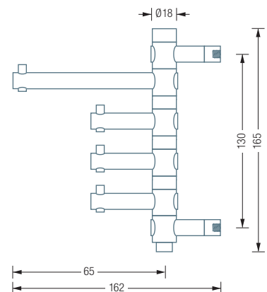
GH4-2 Seitenansicht:
