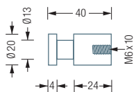
HN20-40 Seitenansicht:
