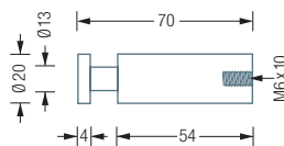
HN20-70 Seitenansicht:
