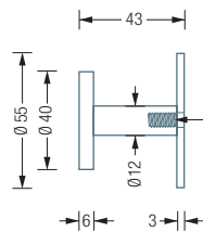
HA3-R55S55 Seitenansicht:
