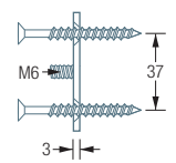
R55VN Seitenansicht:
