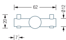
H18-50D Frontansicht:
