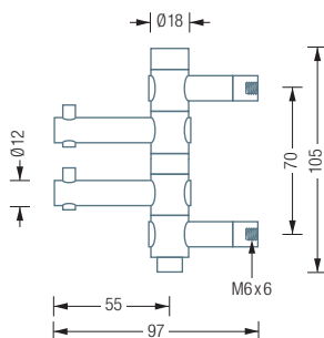
GH2 Seitenansicht:
