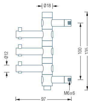
GH3 Seitenansicht:
