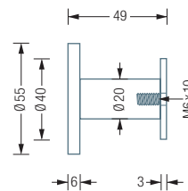
Wandmontage mit Rosette:
