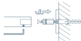
Wandmontage mit Senkhülse und Rosette:
