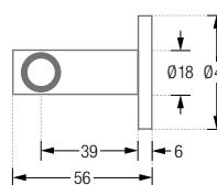
HG18-50DK45-B Seitenansicht:
