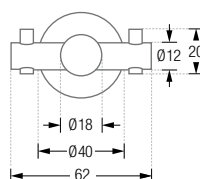
H18-50DR40-B Frontansicht:
