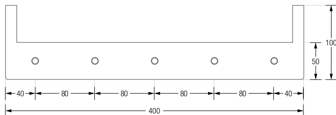
TG5-B Frontansicht:
