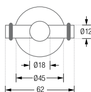
HG18-50DK45-B Frontansicht:
