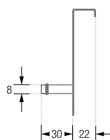
TG3-B/TG5-B Seitenansicht:
