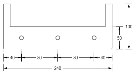
TG3-B Frontansicht:
