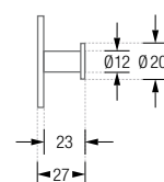
HL3H12S-B/HL5H12S-B Seitenansicht:
