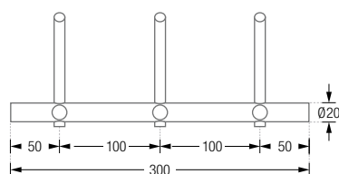
HLS3H-B Frontansicht:
