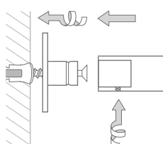
Montage H18-50R40-B:
