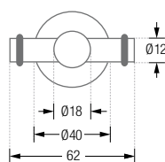
HG18-50DR40-B Frontansicht:
