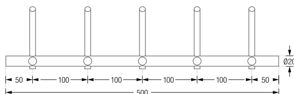
HLS5H-B Frontansicht:
