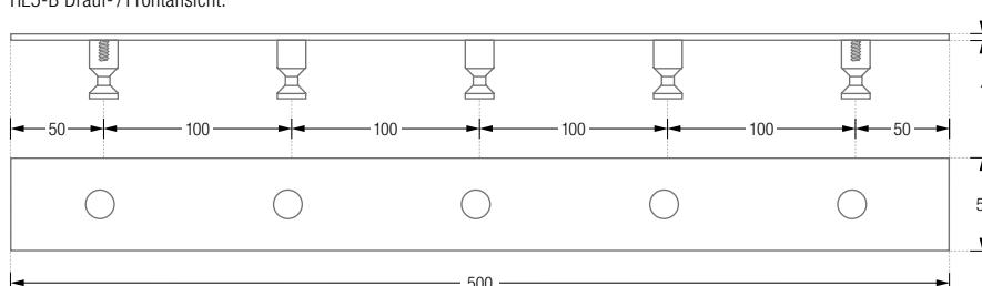
HL5-B Drauf- / Frontansicht:
