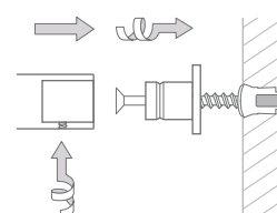
Montage H20-55-B:
