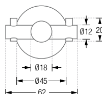
H18-50DK45-B Frontansicht:
