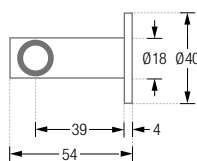
HG18-50DR40-B Seitenansicht:
