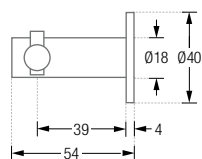
H18-50DR40-B Seitenansicht:
