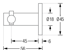
H18-50DK45-B Seitenansicht:
