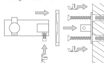
Montage H18-50DR40-B:
