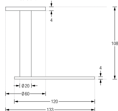
VRH2 Draufsicht:
