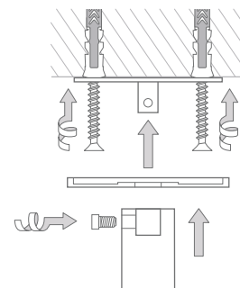
Montage VRH2 mit zweiteiliger Rosette:
