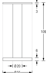
VRH1 Draufsicht:
