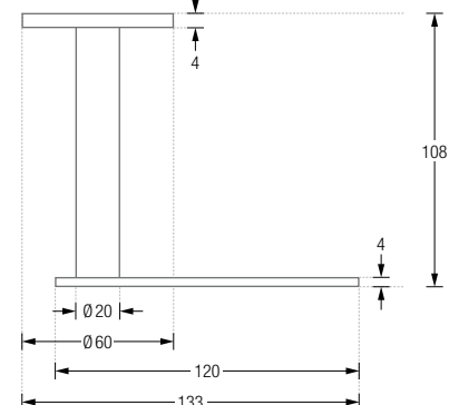
VRH2 Draufsicht:
