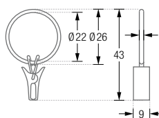
RG26C Front- /Seitenansicht:
