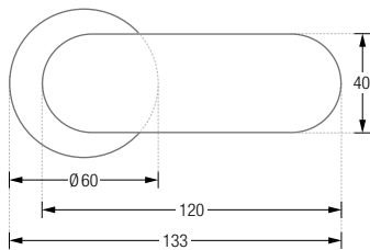
VRH2 Frontansicht:
