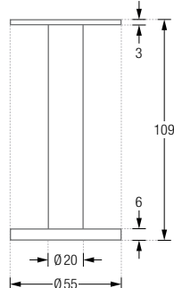
VRH1 Draufsicht:
