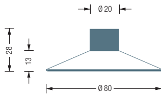
TSB80-13 Seitenansicht:
