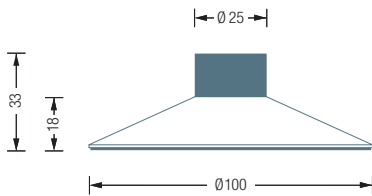
TSB100-18 Seitenansicht:
