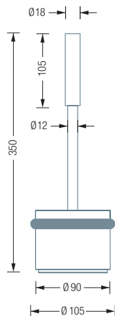
TSB90-75G275:
