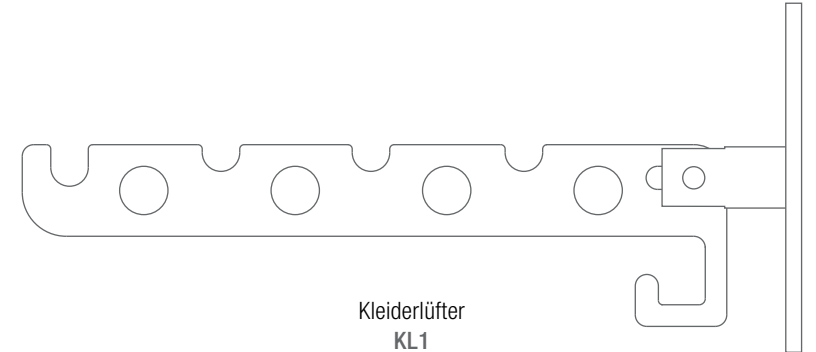
Klapphaken KH
