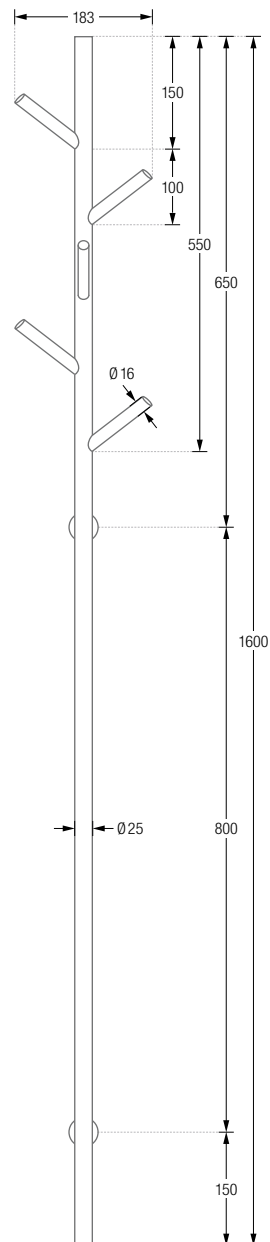
GSTR-W-B Seitenansicht:
