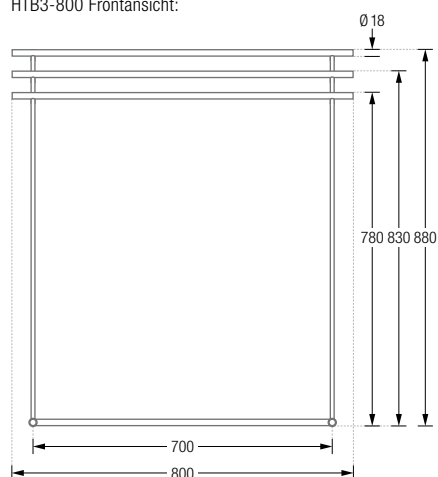
HTB3-800 Frontansicht:
