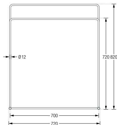
HTB2K-700 Frontansicht:
