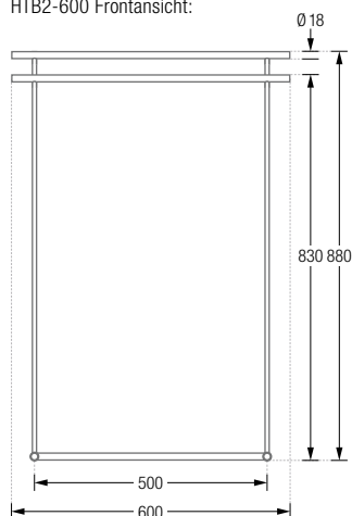
HTB2-600 Frontansicht:
