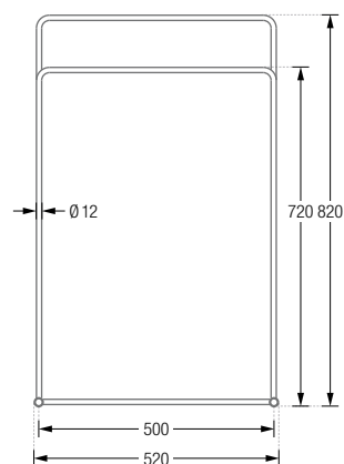
HTB2K-500 Frontansicht:
