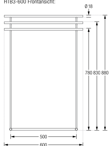
HTB3-600 Frontansicht:
