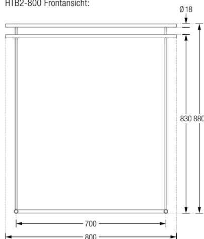
HTB2-800 Frontansicht:
