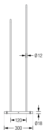
HTB3-600/800 Seitenansicht:
