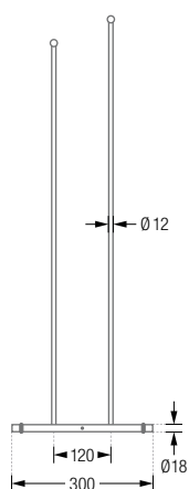
HTB2-600/800 Seitenansicht:
