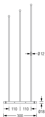
HTB3-600/800 Seitenansicht:
