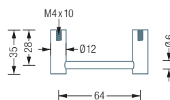
BG6-288E Draufsicht:
