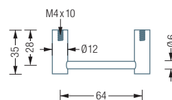
BG6-288E Draufsicht:
