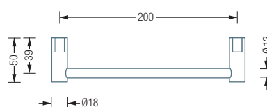
BG12-900E Draufsicht:
