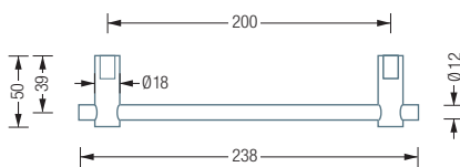
BG12-238 Draufsicht:
