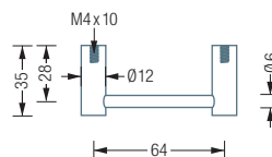
BG6-288E Draufsicht:
