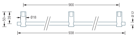
BG12-938 Draufsicht:
