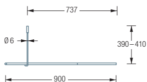
DSB500-900 Seitenansicht:
