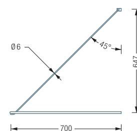
DSU1700-700W Seitenansicht:
