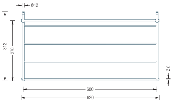
G1-600 / 1200 / 1800 Seitenansicht:
