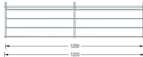
G1-1200 Draufsicht:
