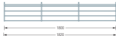
G1-1800 Draufsicht:
