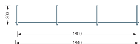
G3-1800 Draufsicht:
