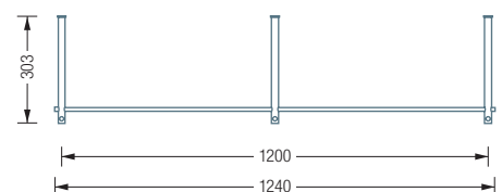
Ablage G3-1200 G/H/CDF/CDFS Draufsicht:
