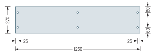
Ablage G3-1200 G/H/CDF/CDFS Draufsicht:
