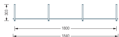
G3-1800 Draufsicht:
